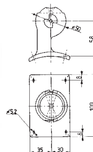
36031300498 Pied de mât tournant pour profils F32C et F49C. Rotating mast step for profiles F32C and F49C.
